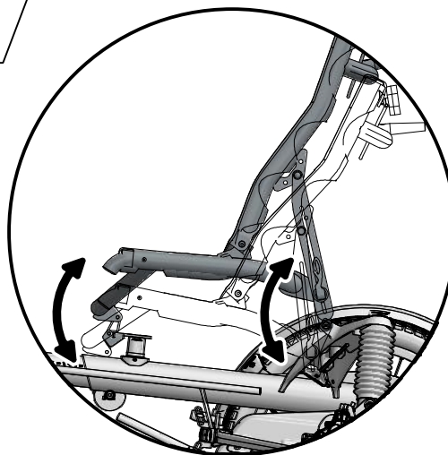
Choisir la hauteur du siège
